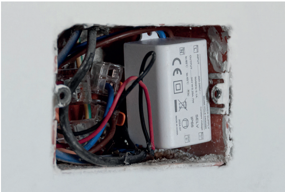
026.330 Power supply that can be inserted inside built-in boxes 026.330 Alimentatore inseribile all'interno di scatole da incasso 026.330 Netzteil zum Einbau in Einbaudosen 026.330 Alimentation pouvant être insérée dans des boîtes à encastrer
